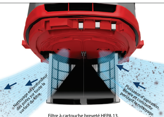
Filtre à cartouche breveté HEPA 13.
